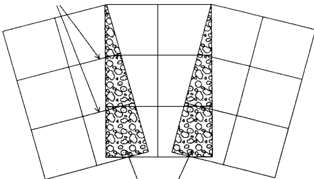
Rys. 11. Materace gabionowe nieprzepuszczalne i półprzepuszczalne
