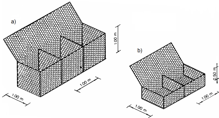
Rys. 1. Przykład gabionów w postaci prostopadłościennych koszów siatkowych Kosz gabionu trzykomorowy 3,0 x 1,0 x 1,0 m Kosz gabionu dwukomorowy 2,0 x 1,0 x 0,5 m
