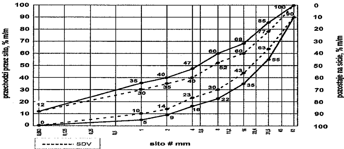
Rysunek 1. Mieszanka niezwiązana 0/63 do warstw podbudowy pomocniczej.
