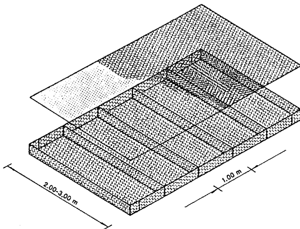
Rys. 8. Umocnienie skarpy matercami gabionowymi, na które przymocowuje się przykrycie siatką z rolki
