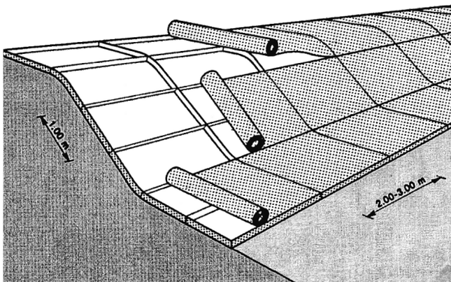
Rys. 8. Umocnienie skarpy matercami gabionowymi, na które przymocowuje się przykrycie siatką z rolki
