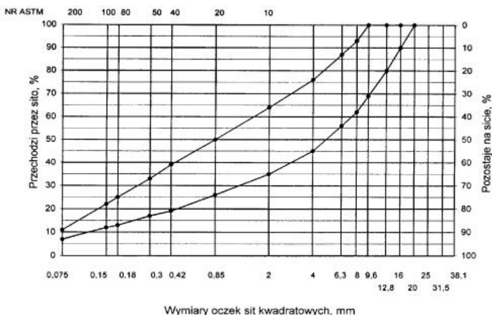
Rysunek 1. Krzywe graniczne uziarnienia mieszanki mineralnej BA
